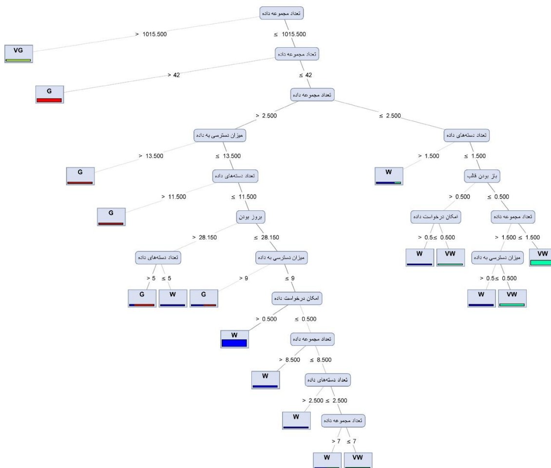
شکل ۱۸. درخت تصمیم
