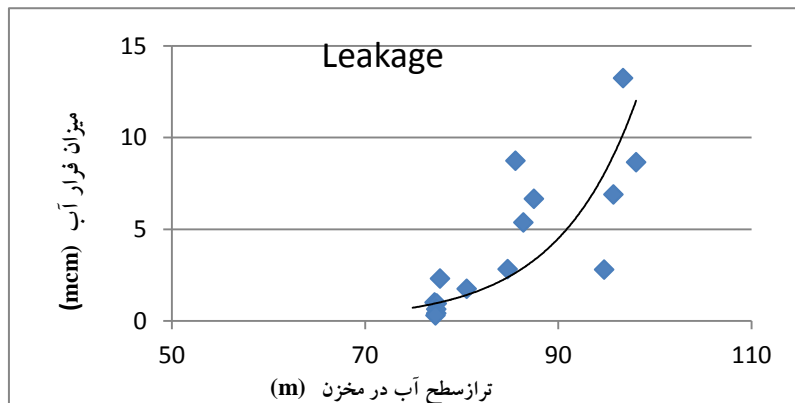
شکل ۴. نمودار نتایج سطح تراز آب و فرار آب
