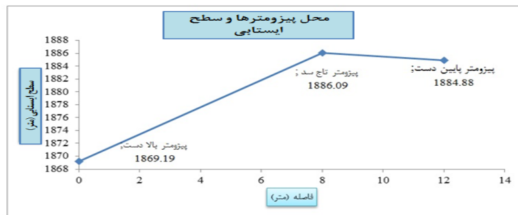
شکل ۷. رفتار نامتعارف مشاهده‌های پیزومتریک در بخشی از سد
