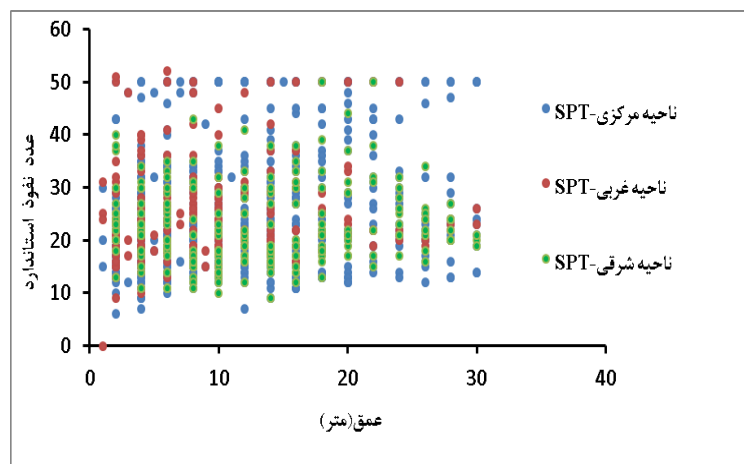
شکل ۱۰. بررسی تغییرات عدد نفوذ استاندارد در نواحی سه‌گانه در زیر پهنه شهر کرمان
