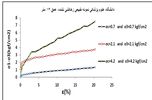
شکل ۲۲. منحنی‌های تنش- کرنش محوری نمونه‌های طبیعی زهکشی نشده، دانشگاه علوم پزشکی کرمان عمق ۱۴،۴۵-۱۴ متر
