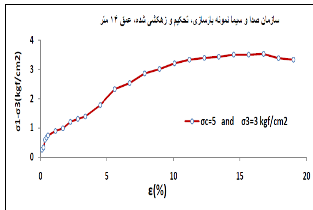
شکل ۱۳. منحنی تغییرات تنش - کرنش محوری نمونه بازسازی و زهکشی شده، سایت سازمان صدا و سیمای مرکز کرمان و سیمای عمق ۱۴-۱۴،۴۵ متر
