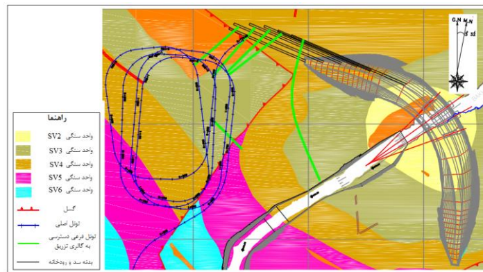
شکل ۱. پلان جانمایی تونل دسترسی حلزونی، سایر دسترسی‌ها به گالری‌های تزریق و زمین‌شناسی محدوده ساختگاه و مسیر تونل حلزونی سد و نیروگاه بختیاری [۷]
