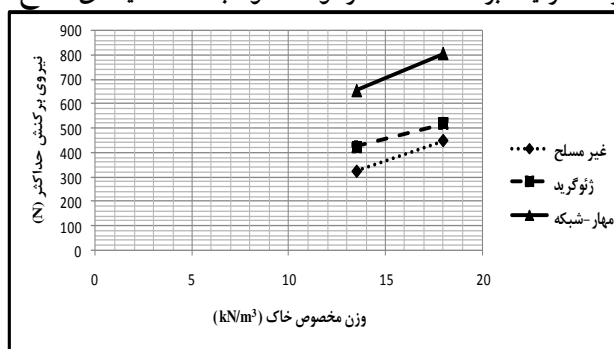
شکل ۱۸. تغییرات ظرفیت بر خاست لوله مدفون با تغییر وزن مخصوص ماسه اثر قطر لوله (D)
