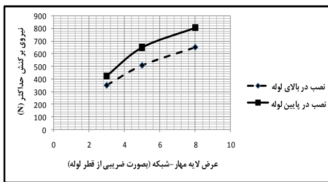
شکل ۱۶. نحوه تغییرات مقاومت بر خاست لوله با عرض لایه مهاری- شبکه به صورت نصب در بالا و پایین لوله
