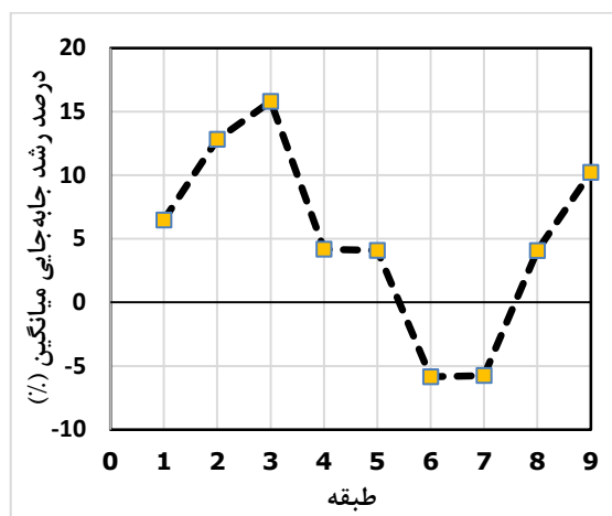
شکل ۱۷. درصد رشد جابه‌جایی نسبی طبقات سازه ۹ طبقه در اثر شیب مورد نظر نسبت به حالت
