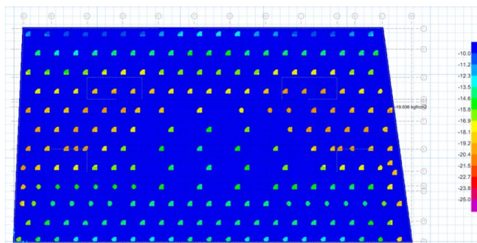
شکل ۵ پلان جانمایی و تنش‌های وارد بر ستون‌های جت‌گروت در طرح اولیه ( \text{kg/cm}^2 )
