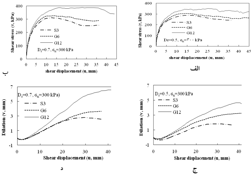
شکل ۳: رفتار برشی و اتساعی و انقباضی خاک تحت سربار ۳۰۰ کیلوپاسکال با دانسیته نسبی (الف) (ب و ج) ۵۰ درصد و (د) ۷۰ درصد
