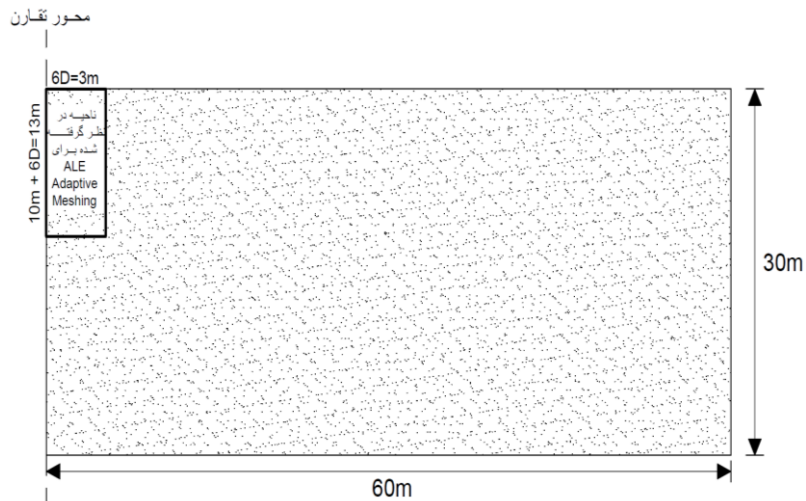
شکل ۴. ابعاد خاک مسئله و ناحیه در نظر گرفته شده برای مش‌بندی انطباقی لاگرانژی-اویلری اختیاری
