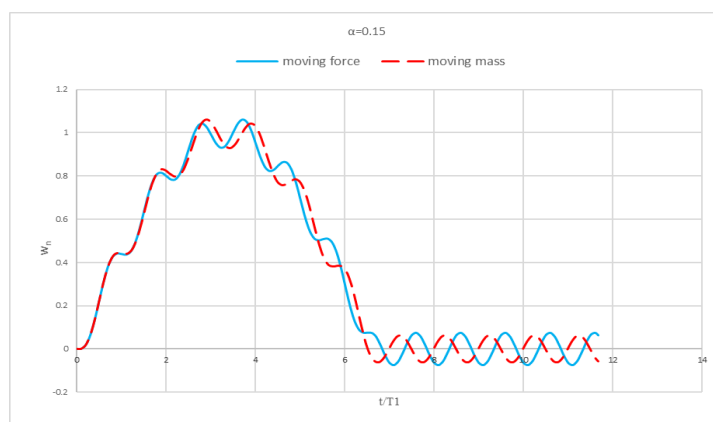
شکل ۹. تاریخچه تغییر مکان دینامیکی وسط دهانه به تغییر مکان استاتیکی نظیر به ازای پارامتر سرعت \alpha = 0.15
