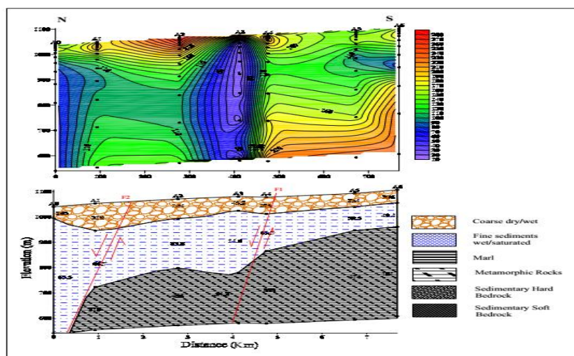
شکل ۷. مقطع مقاومت ظاهری (شکل بالا) و مقاومت حقیقی همراه با نیم‌رخ زمین‌شناسی (شکل پایین) در مسیر پروفیل A-A [۵]
