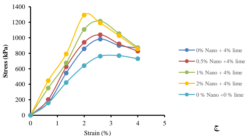
شکل ۳. مقاومت تک‌محوری خاک همراه با درصد‌های مختلف افزودنی آهک و نانورس (الف) نمونه‌ها بدون افزودنی آهک با ۲ درصد (ب) نمونه‌ها با ۴ درصد (ج) نمونه‌ها با ۴ درصد آهک
