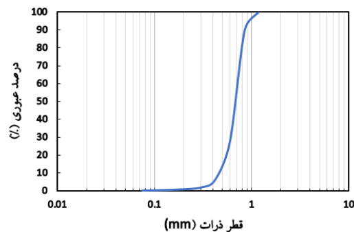
شکل ۱. نمودار دانه‌بندی مصالح مصرفی
