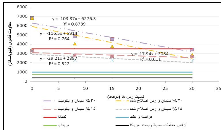
شکل ۳. تغییرات مقاومت فشاری آزاد با نسبت‌های مختلف رس معمولی و اصلاح شده با زمان عمل‌آوری ۲۸ روز
