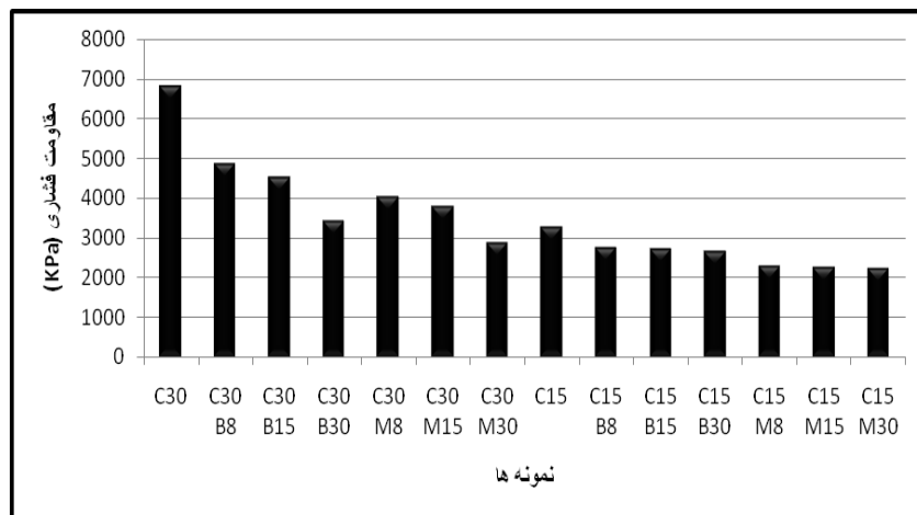
شکل ۲. مقاومت فشاری آزاد نمونه‌های آلوده به فنل با استفاده از رس معمولی و اصلاح شده
