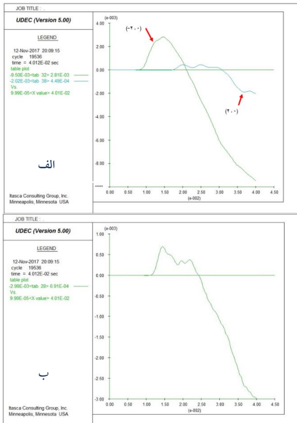
شکل ۱۱. تاریخچهٔ زمانی جابه‌جایی‌های افقی (الف) در نقاط شاهد (۲، ۰) و (۰، ۲) روی دیوارهٔ سمت چپ و راست رمپ، (ب) در نقطه شاهد (۲/۱، ۰) روی سقف در مدت زمان ۴۰ میلی ثانیه از اعمال بار دینامیکی
