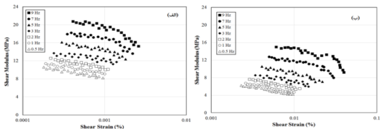
شکل ۱۳. تغییرات مدول برشی با کرنش برشی در فرکانس‌های مختلف بارگذاری تحت بارگذاری مثلثی و شتاب ورودی الف) 0.1g ، ب) 0.3g
