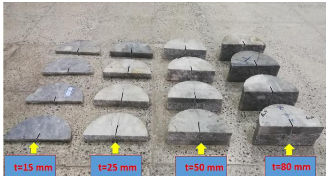
شکل ۴. نمونه‌های SCB از جنس سنگ مرمریت قروه با شعاع یکسان اما ضخامت‌های مختلف
