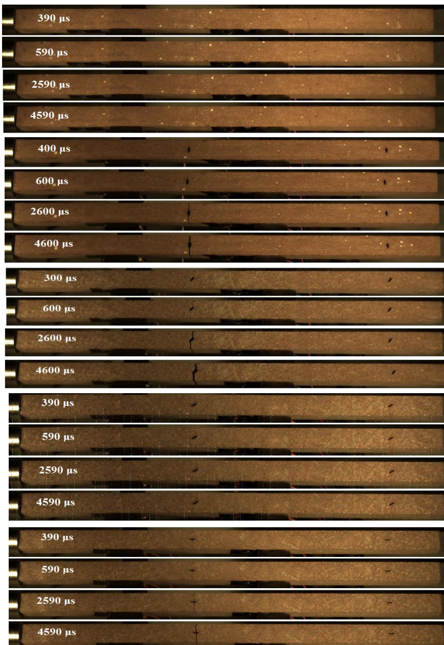
شکل ۶. نحوه گسیختگی اسپالینگ نمونه‌ها در آزمون بارگذاری دینامیکی
