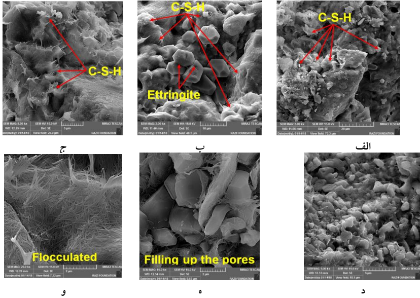
شکل ۶. ریزساختارهای نمونه خاک شماره ۵ دو (MCS)
