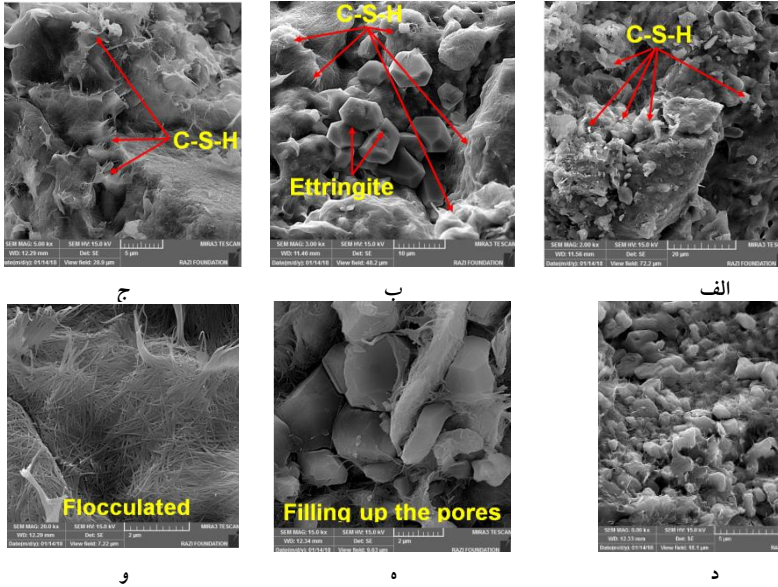
شکل ۶. ریزساختارهای نمونه خاک شماره ۵ (MCS)
