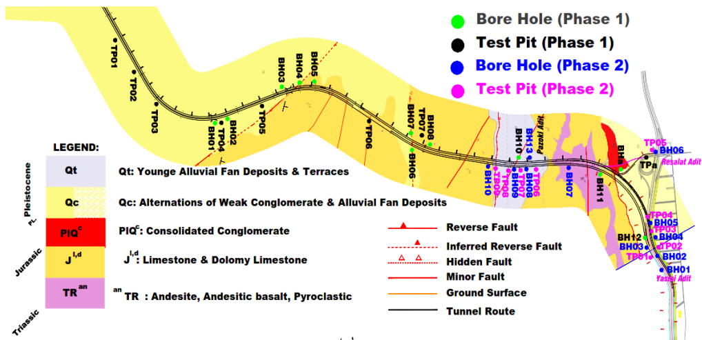
شکل ۱. الف) نقشه زمین شناسی و گسل های شهر تهران، ب) پلان زمین شناسی و موقعیت گمانه ها و چاهک های شناسایی مسیر تونل [۲۱]
