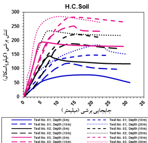
شکل ۱۲. نتایج آزمون‌های برش برجا در عمق‌های مختلف
