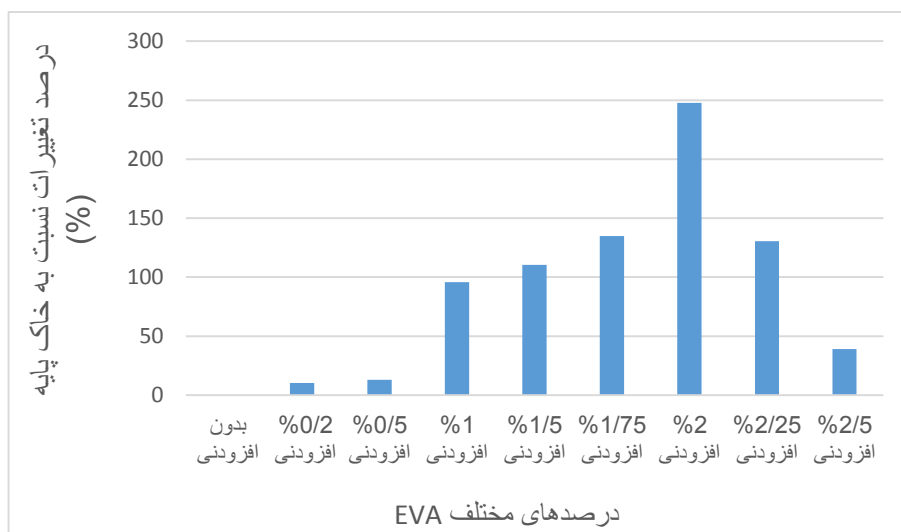
شکل ۱۵- درصد تغییرات مقدار CBR برای درصدهای مختلف افزودنی نسبت به خاک پایه برای حالت نمونه سست
