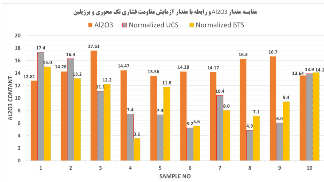
شکل ۱۵- مقایسه درصد Al 2 O 3 با مقاومت فشاری تک محوری و برزیلین (مقدار مقاومت ها نرمال شده اند).
