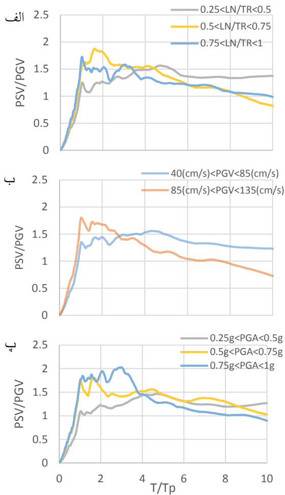
شکل ۶- طیف پاسخ شبه سرعت نرمال دوسویه با معیار پرئود غالب T_p ، (با نماد (BNPVS(T_p)) )
