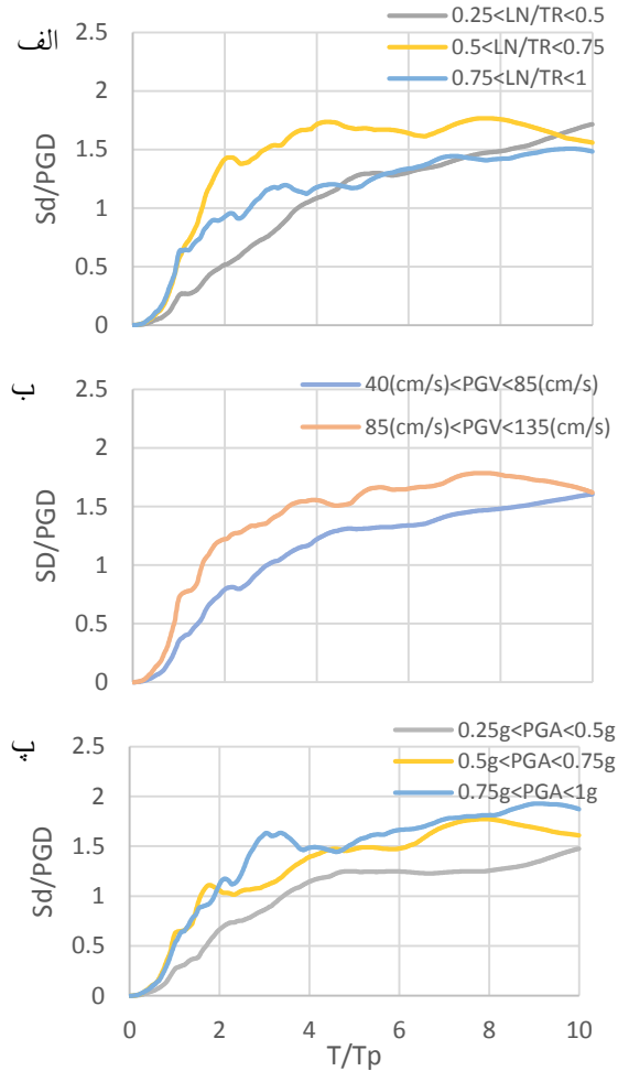
شکل ۵- طیف پاسخ جابجایی نرمال دوسویه با معیار پرئود غالب T_p ، (با نماد (BND(S(T_p)) )
