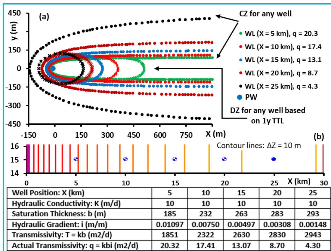
شکل ۱۳. (a) حریم آبرفتی و حریم تخلیه برای موقعیت چاه در جهت جریان از مرز تخلیه تا مرز تقسیم. (b) موقعیت چاه‌ها در عرض ۱۵ کیلومتری. خطوط زمان گذر ۱ ساله هستند.
