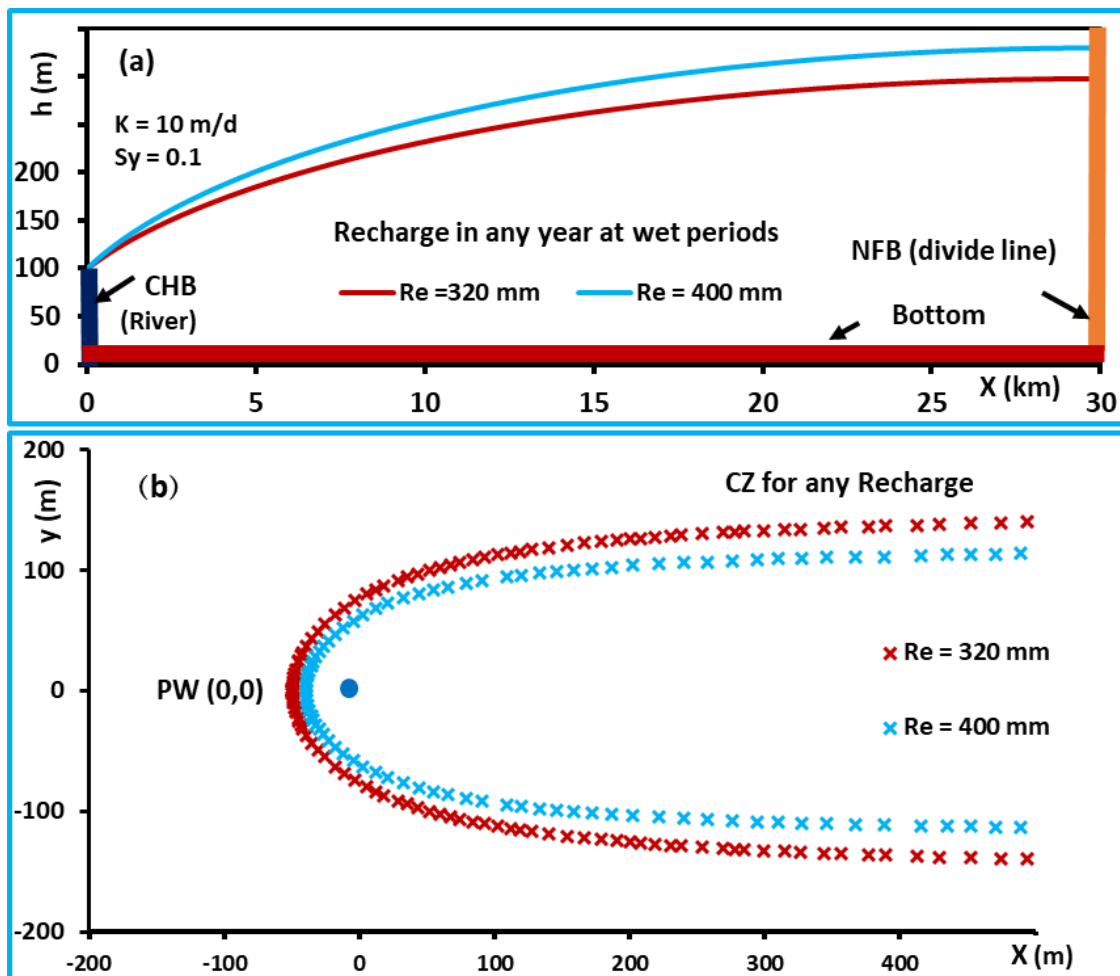
شکل ۱۵. اثر نسبت تخلیه به تغذیه بر حریم آبیگر در چاه مرکزی آبخوان. شکل تغییر حریم آبیگر چاهی در مرکز یک آبخوان را نشان می‌دهد که سطح تراز آن از طریق چاههایی که به طور مناسب در کل آبخوان جانمایی شده‌اند تنزل یافته است. مقدار تخلیه‌ی کل چاه‌ها معادل ۸۰ میلی‌متر از کل تغذیه‌ی آبخوان بوده است.
