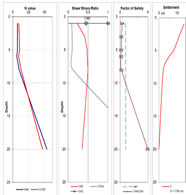
شکل ۱۳. شرایط عدد SPT، نسبت تنش برشی، وضعیت روانگرایی و نشست در گمانه شماره ۳ به روش سید و ادریس Fig. 13. The Conditions of SPT number, shear stress ratio, and liquefaction and settlement condition in borehole No.3 by Seed and Idriss method
