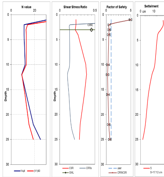
شکل ۱۲. شرایط عدد SPT، نسبت تنش برشی، وضعیت روانگرایی و نشست در گمانه شماره ۲ به روش سید و ادریس Fig. 12. The Conditions of SPT number, shear stress ratio, and liquefaction and settlement condition in borehole No.2 by Seed and Idriss method
