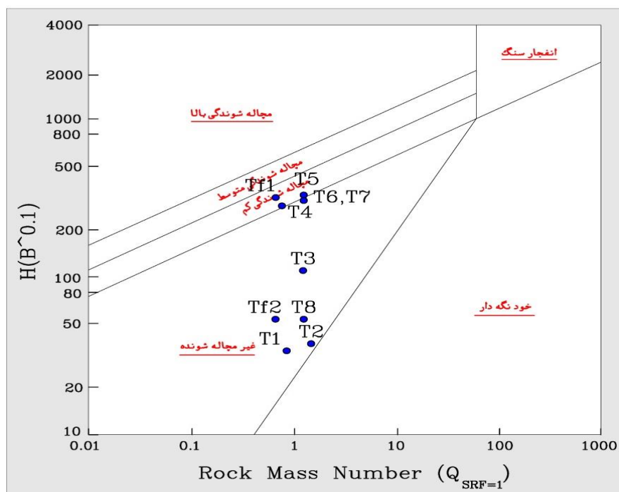
شکل ۷. وضعیت بخش‌های مختلف دارای پتانسیل لهیدگی بر اساس نمودار گوئل و همکاران (Goel et al., 1995) Fig. 7. The status of different unite with squeezing potential based on the diagram of Goel et al. (1995)
