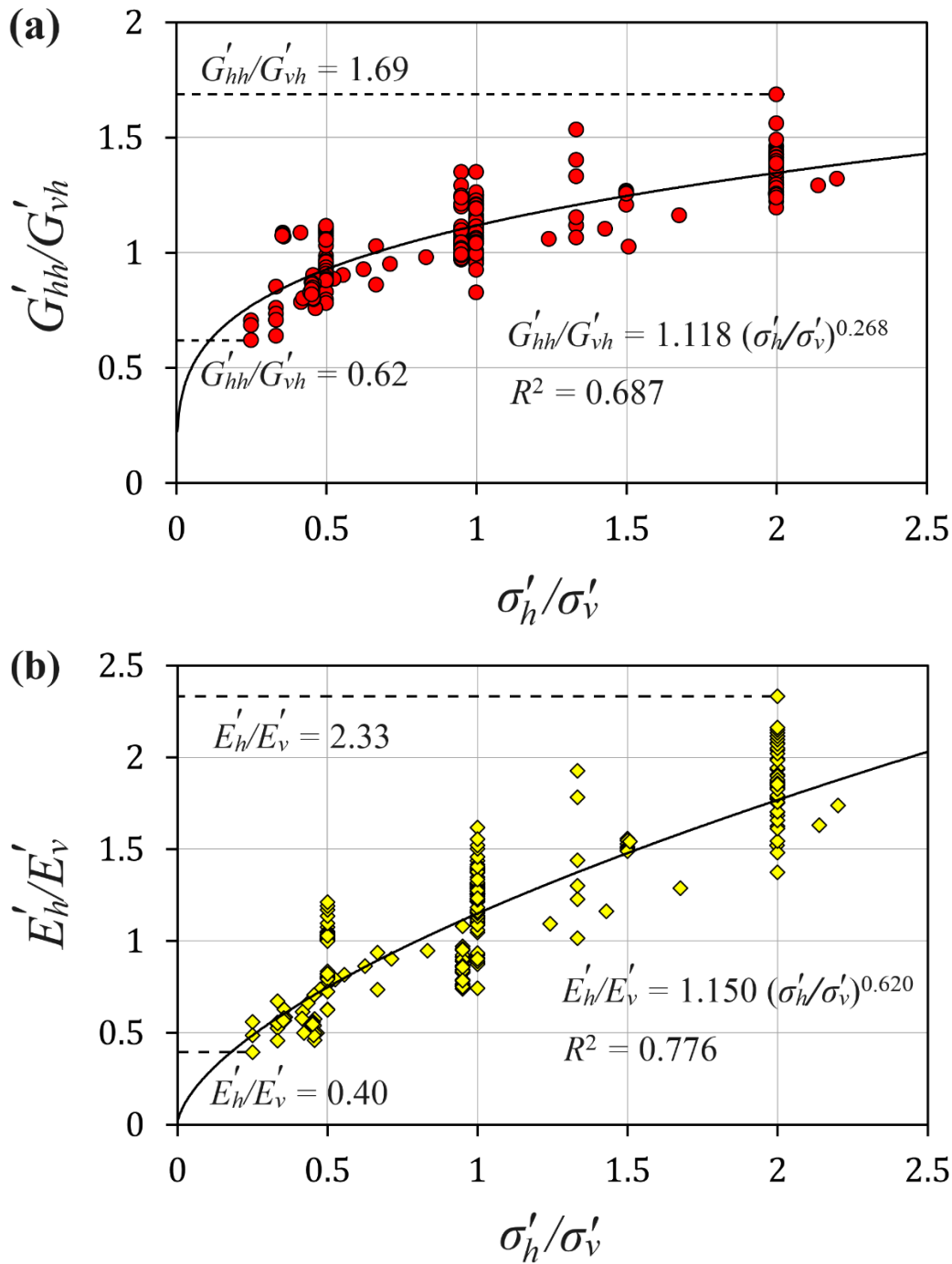
شکل ۱. مدل تغییرات نسبت‌های ناهمسانگردی مدول برشی G'_{hh}/G'_{vh} و (a) مدول برشی G'_{hh}/G'_{vh} ، و (b) مدول یانگ E'_h/E'_v در برابر نسبت تنش \sigma'_h/\sigma'_v در خاک‌های غیر چسبیده
