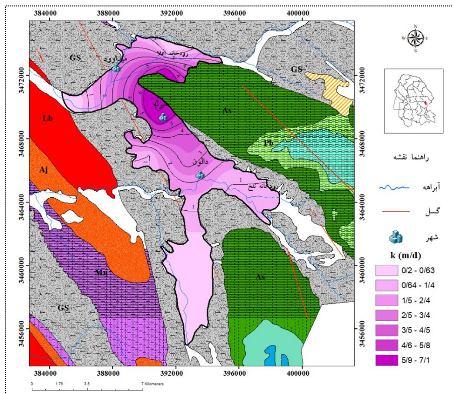
شکل ۶. نقشه پهنه‌بندی هدایت هیدرولیکی دشت دالون-میداود (روش آزمون پمپاژ)
