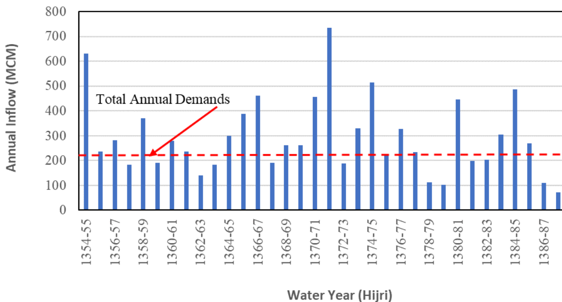
شکل ۲. آبدهی‌های سالانه ورودی به سد جره (محور افقی سال آبی بر حسب تقویم هجری شمسی و محور عمودی آبدهی سالانه بر حسب میلیون متر مکعب است)
