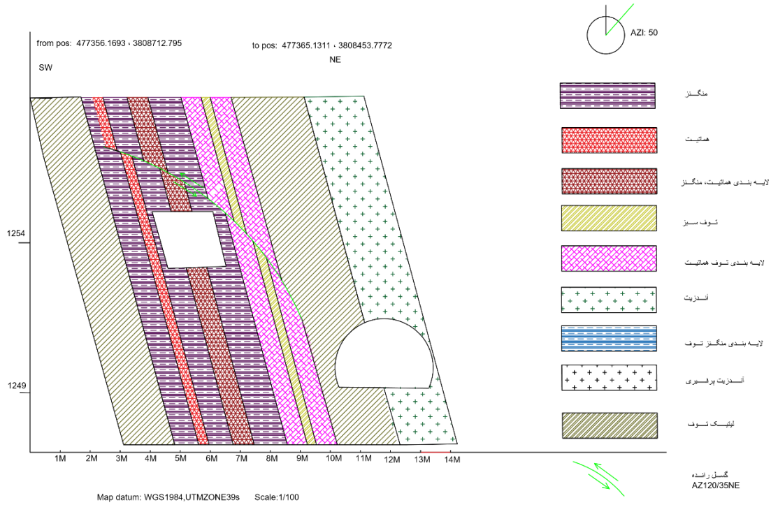
شکل ۳. مقطع عرضی از واحدهای سنگی و حفریات، در قسمت دوم محدوده ( همراه گسل). Fig. 3. Cross-section of stone units and excavations, in the second part of the range (along the fault).
