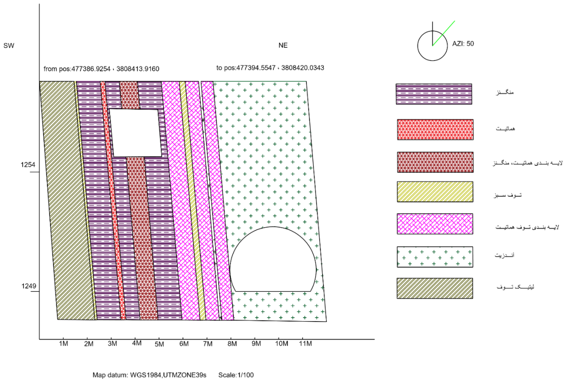
شکل ۲. مقطع عرضی از واحدهای سنگی و حفریات، در قسمت اول محدوده ( بدون گسل). Fig. 2. Cross-section of stone units and excavations, in the first part of the range (without faults)
