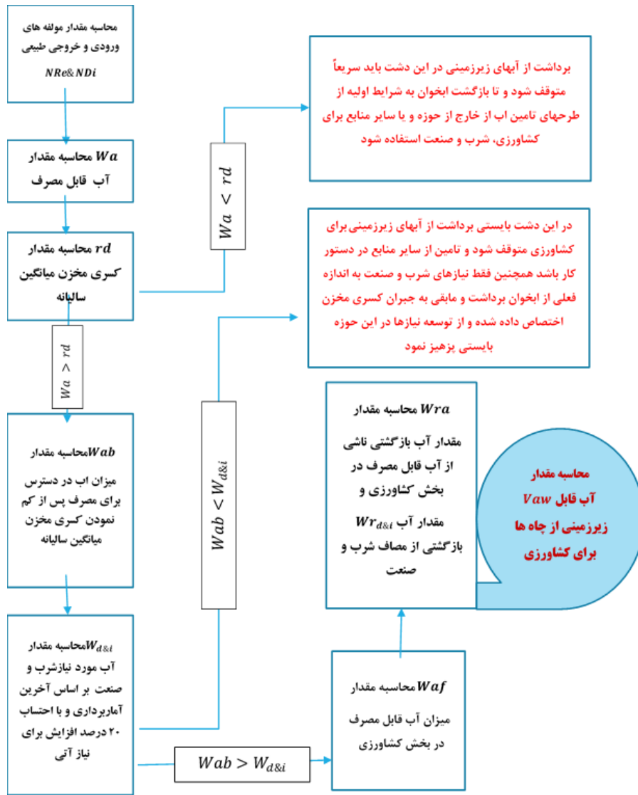
شکل ۱. فلوجارت کاربردی برای روش پیشنهادی محاسبه آب زیرزمینی قابل برنامه‌ریزی
