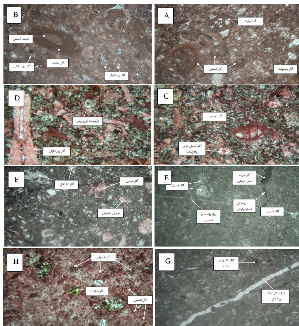
شکل ۴. A- سنگ با زمینه اسپارایتی و آسترولینا در نمونه رنگ آمیزی شده توسط آلizarin، با بزرگنمایی AE4 (PPL)، B- آثار جلبک در نمونه رنگ آمیزی شده توسط آلizarin، با بزرگنمایی AE4 (XPL)، C و D- آثار دولومیت در نمونه رنگ آمیزی شده توسط آلizarin، با بزرگنمایی EA10 (XPL) و دولومیت لوزوجهی با بزرگنمایی EA4 (PPL)، E- درزه های استیلولیتی و ریز درزه های کلسیتی، بزرگنمایی AE4 (XPL)، F- آثار حفرات خالی، G- شکستگی فاقد پرشدگی و آثار کانی های اپاک با بزرگنمایی AE4 (PPL)، H- گلوکونیت در نمونه رنگ آمیزی شده توسط آلizarin، با بزرگنمایی EA4 (PPL).
