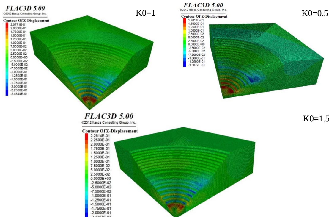
شکل ۸. کنطور جابه‌جایی‌ها در راستای Z در سناریوی سوم برای نسبت‌های تنش افقی به قائم ۱/۵ و ۰/۵. Fig. 8. Displacement contours in the Z direction in Scenario 3 for horizontal-to-vertical stress ratios of 0.5, 1, and 1.5
