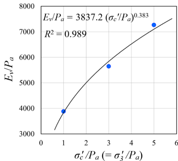
شکل ۷. برازش منحنی نسبت E_v/P_a بر حسب \sigma'_c/P_a (= \sigma'_3/P_a) به منظور تعیین ثابت‌های K و n مربوط به ستون خاک در ساختگاه آزمایشی
