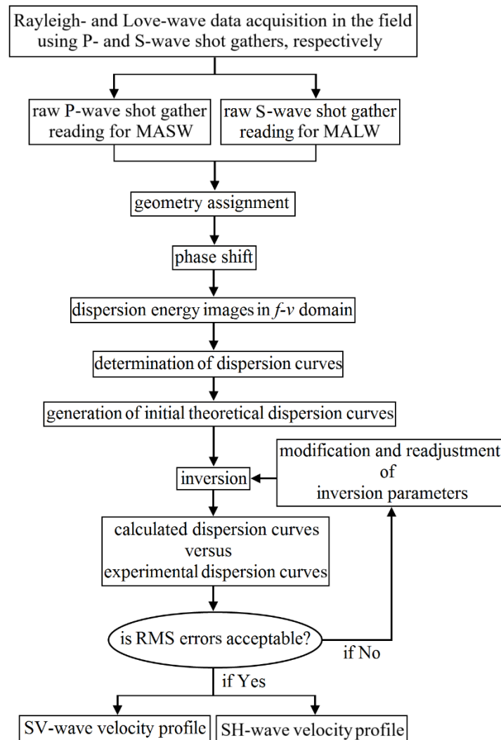
شکل ۵. فلوچارت مراحل برداشت، پردازش و معکوس‌سازی داده‌ها با استفاده از روش‌های MASW و MALW در این مطالعه برای استخراج پروفیل‌های سرعتی موج SV و SH
