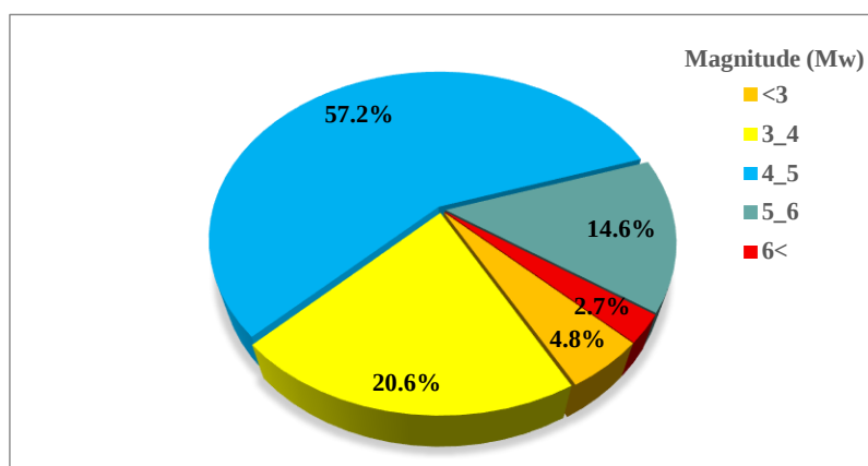
شکل ۴. فراوانی زمین‌لرزه‌ها در بازه‌های مختلف بزرگای در پیرامون ساختگاه (بازه زمانی ۱۹۰۰ تا ۲۰۲۲) Fig. 4. Frequency of earthquakes at different magnitude intervals around the site (time period from 1900 to 2022)
