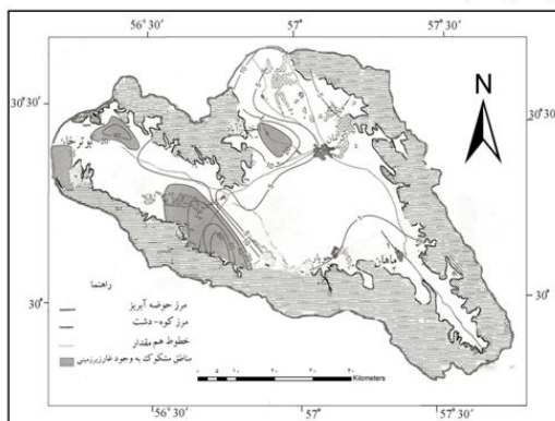
شکل ۹. نقشه مقادیر نمایه انحلال و موقعیت مناطق مشکوک به وجود غار زیرزمینی که با هاشور تیره مشخص شده‌اند
