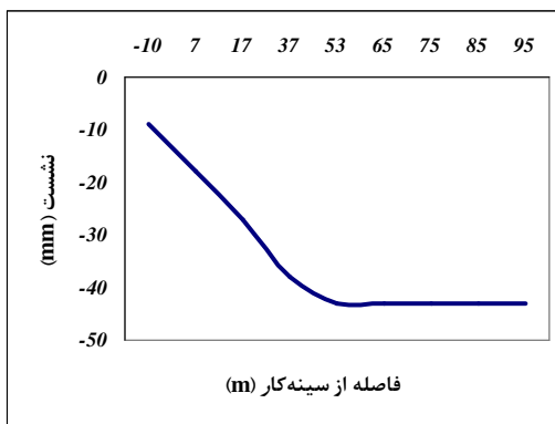
شکل ۷. جابه‌جایی در مقطع طولی تونل طولی در مقطع بررسی شده
