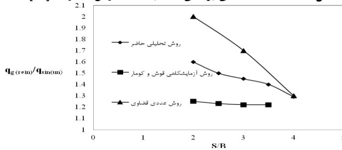
شکل ۷. بررسی تأثیر فاصله بین پی ها بر نسبت ظرفیت باربری پی های اجرا شده نزدیک هم واقع بر خاک مسلح به پی های منفرد واقع بر خاک غیرمسلح از روش های ارائه شده در گذشته و روش ارائه شده در تحقیق حاضر [۶]، [۱۰]
