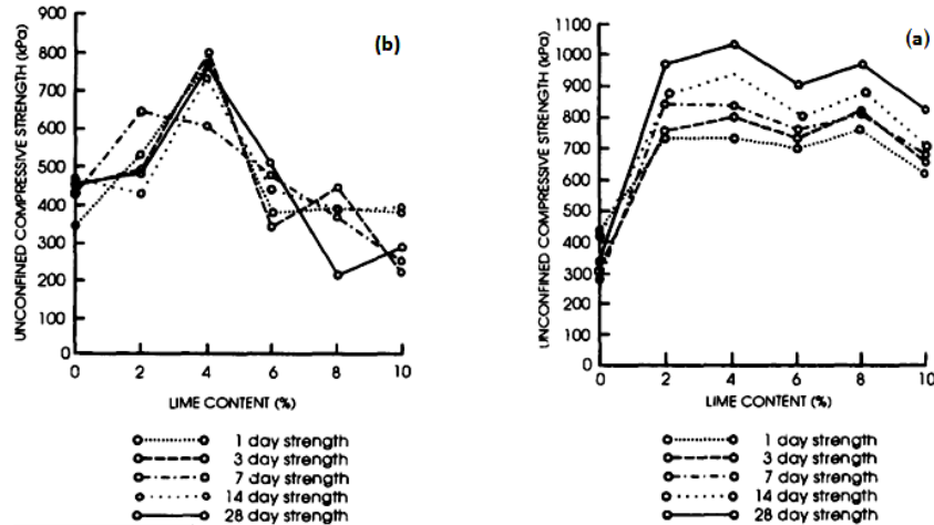
شکل ۱. مقاومت فشاری ساده: (a) کائولینیت، (b) مونتوریلونیت با درصدهای مختلف آهک [۸]
