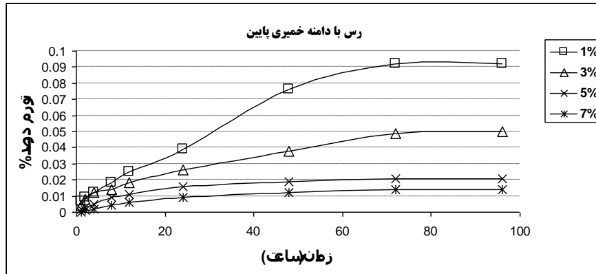
شکل ۱۰. تغییرات درصد تورم با زمان برای درصد‌های مختلف افزودنی سیمان به خاک رس با دامنه خمیری کم
