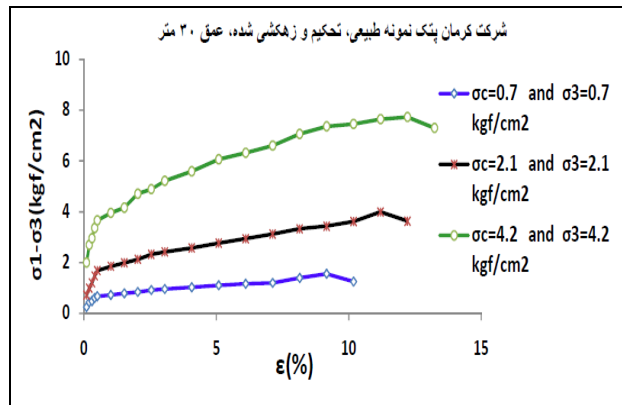
شکل ۱۸. منحنی تغییرات تنش- کرنش محوری نمونه‌های طبیعی زهکشی شده، سایت شرکت کرمان پتک عمق ۳۰، ۳۰، ۴۵ متر
