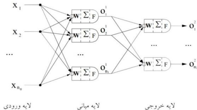
شکل ۴. ساختار شبکه عصبی چند لایه
