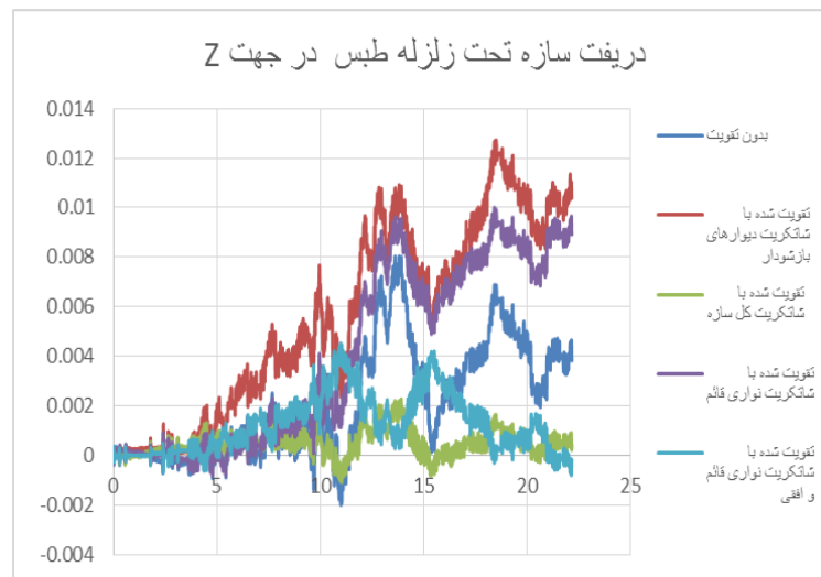
شکل ۱۲. الف) نمودار دریف‌ت سازه تحت زلزله طبرس در جهت Z
