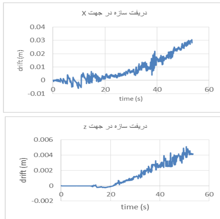
شکل ۱۴. نمودار دررفت سازه تحت زلزله منجیل
