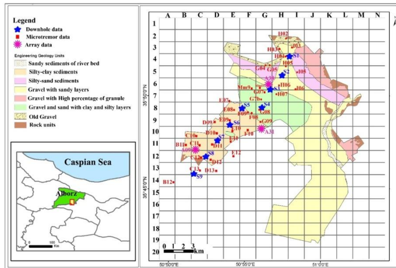
شکل ۳. نقشه زمین‌شناسی مهندسی، موقعیت داده‌های میکروترموورها و داده‌های درون گمانه‌های شهر کرج در بررسی حاضر
