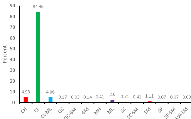
شکل ۵. نسبت فراوانی کلاس‌های خاک بر اساس طبقه‌بندی متحد
