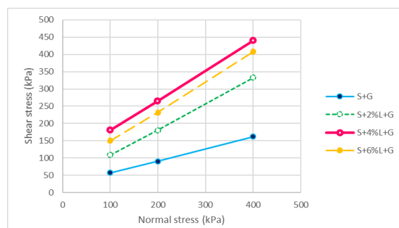
شکل ۱۳. پوش گسیختگی خاک تثبیت شده با درصدهای مختلف آهک و مسلح شده با ژئوگرید ۱۰×۱۰ میلی‌متر بدون المان‌های متقاطع عرضی در درصد رطوبت بالاتر از بهینه
