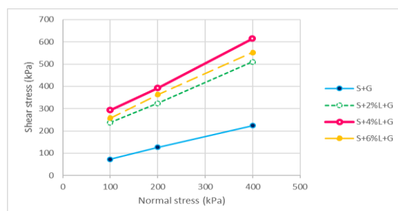
شکل ۱۲. پوش گسیختگی خاک تثبیت شده با درصدهای مختلف آهک و مسلح شده با ژئوگرید ۱۰×۱۰ میلی‌متر بدون المان‌های متقاطع عرضی در درصد رطوبت بهینه
