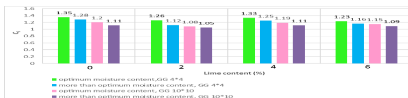
شکل ۲۰. پارامتر C_u برای همه نمونه‌های مسلح شده
