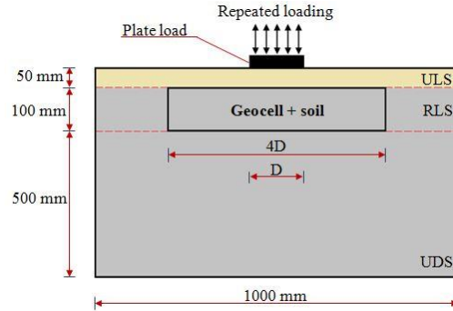
شکل ۵. ابعاد کلی مدل آزمایشگاهی، موقعیت قرارگیری لایه‌های خاکریزی و صفحه بارگذاری
