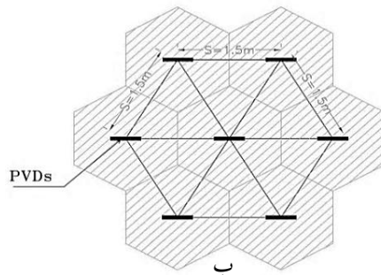
شکل ۶. الف) اجرای زهکش‌های نواری در زیر خاکریزها ب) آرایش زهکش‌ها در پلان
