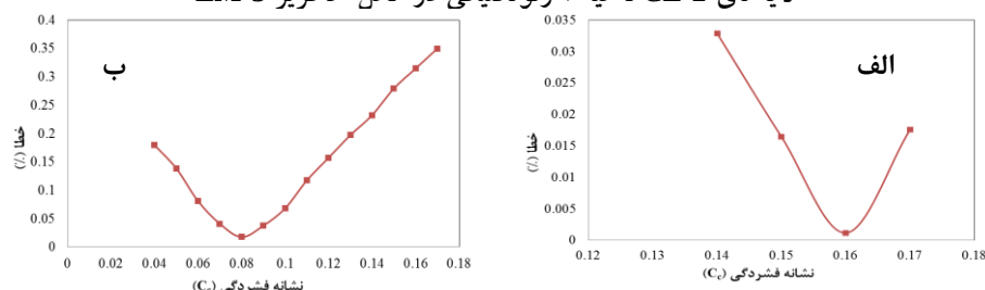
شکل ۲۰. الف) نمودار کمین‌سازی تابع خطا برای پارامتر نشانه فشردگی ( C_c ) در لایه ML ناحیه ۲ ژئوتکنیکی، ب) نمودار کمین‌سازی تابع خطا برای پارامتر نشانه فشردگی ( C_c ) در لایه CL-1 ناحیه ۲ ژئوتکنیکی
