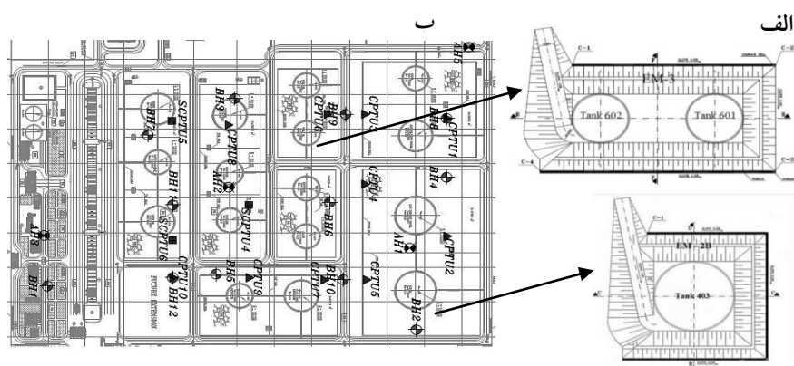
شکل ۷. الف) پلان موقعیت خاکریزهای EM-2B و EM-3، ب) محل گمانه های ناحیه دو و سه ژئوتکنیکی
